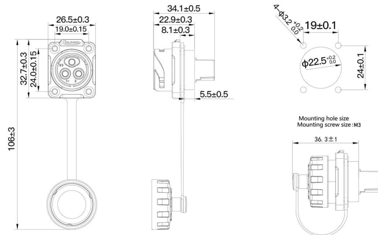
Socket
