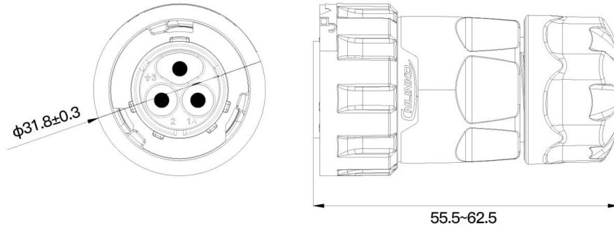
Socket
