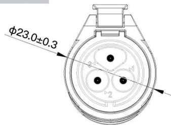
Socket
