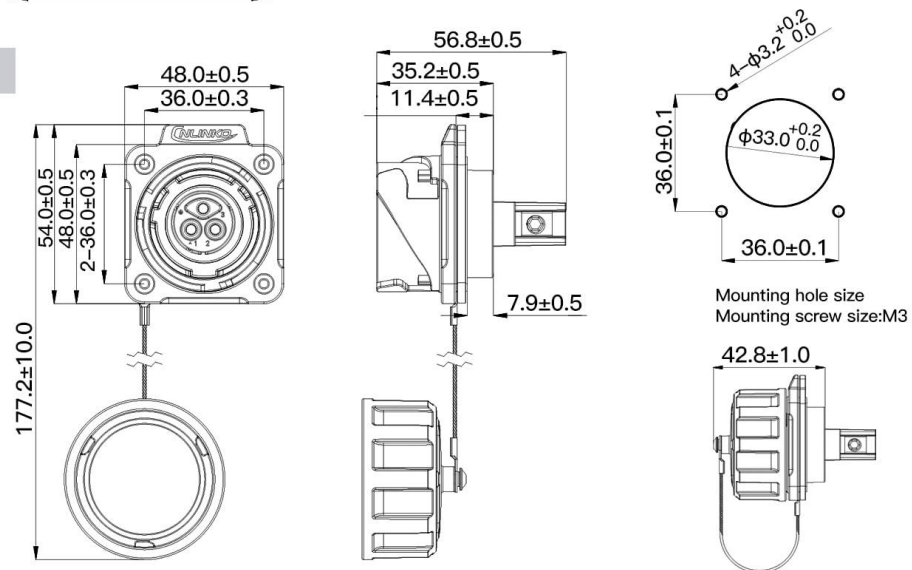
Socket
