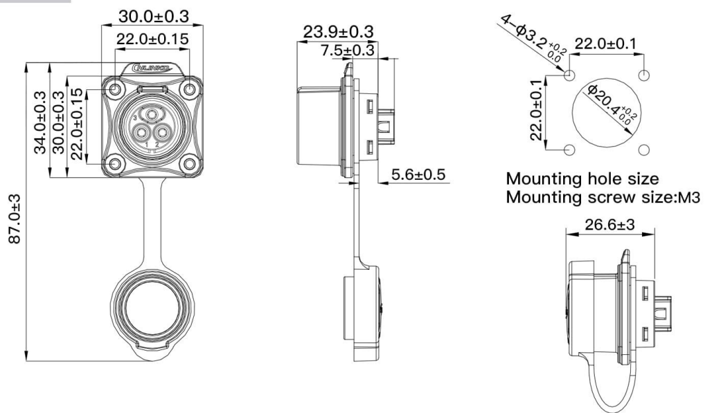
Socket
