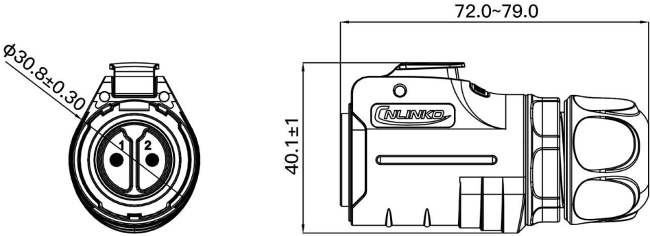
Socket
